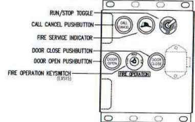
2004-2007 ASME FIRE CABINET SUBPLATE LAYOUT
